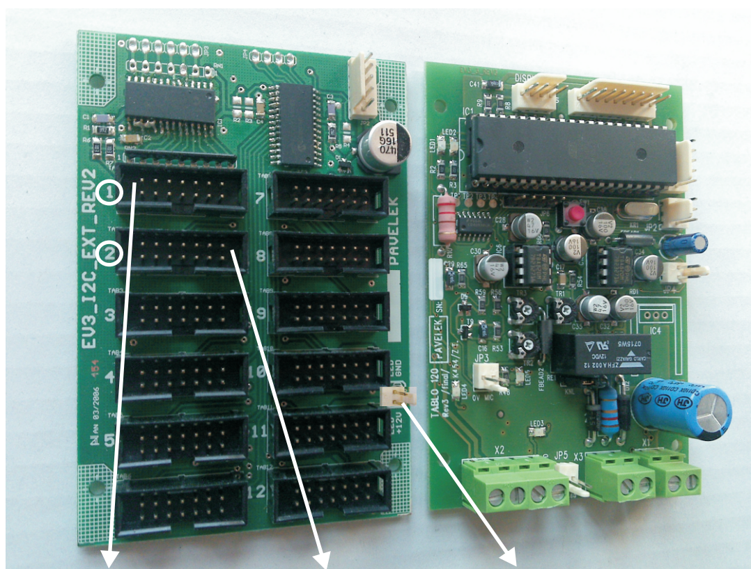
modul komunikace 10 tlač. modul jmenovek konektor na propojení podsvětlení z pohybového čidla 10V=
